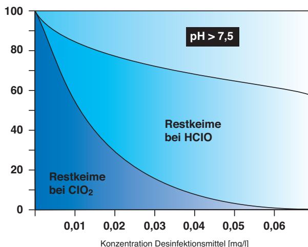
Effektivitätsdiagramm
