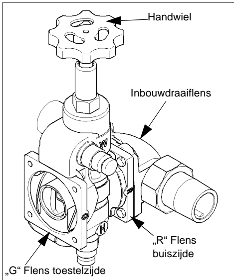
Afb. 5: Drukvereffeningsventiel
