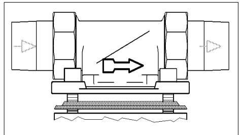
Afb. 4: inbouwdraaiflens
