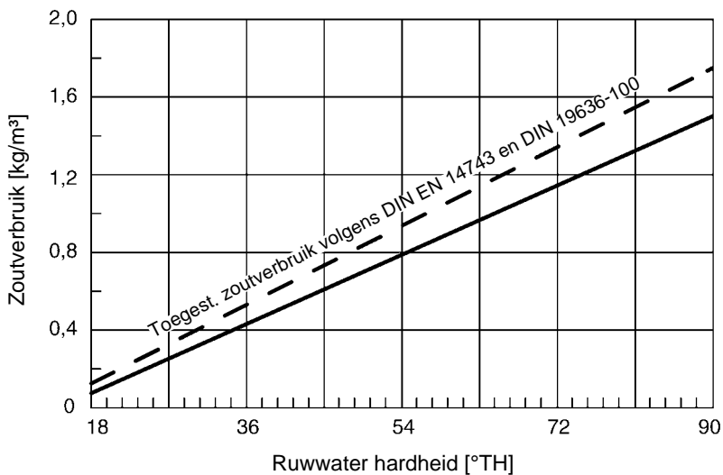
Afb. 16: Zoutverbruik
