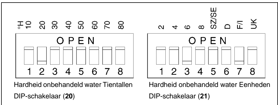
Abb. 10: DIP-schakelaar
