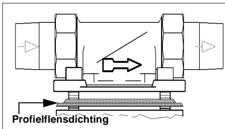
Afb. 9: Inbouwdraaiflens
