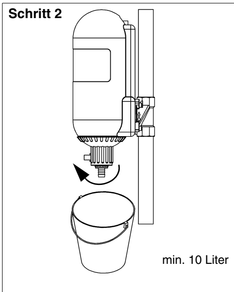
Abb. 7: Vor der Rückspülung den Spülhahn nach vorne drehen. Die Durchströmung des Gerätes wird dadurch unterbrochen.
