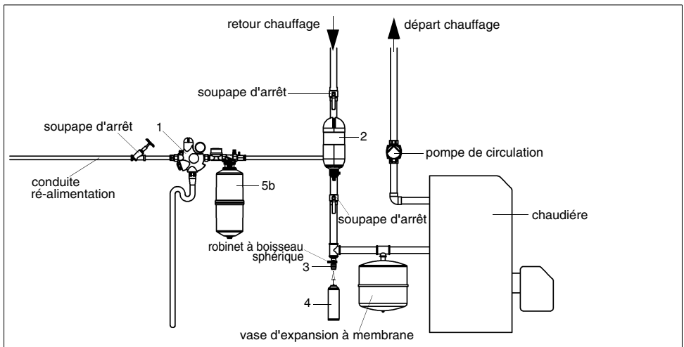
Fig. 3: Schéma JUDO HEIFI-TOP avec dispositif fixe de traitement de l'eau selon VDI 2035
