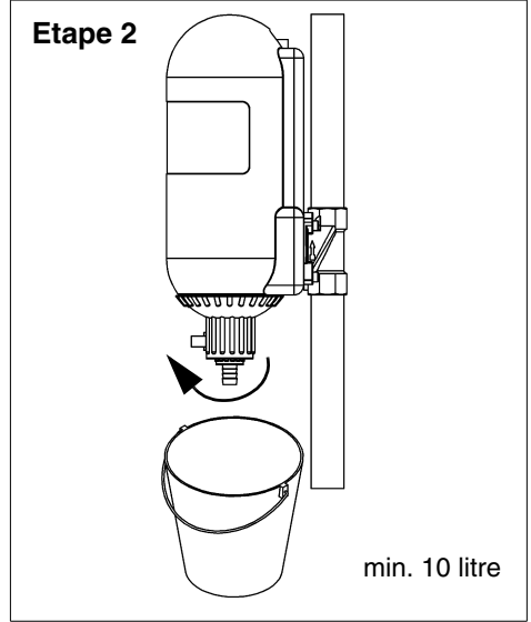
Fig. 8: Avant la performance du rétro lavage il faut tourner le robinet à biseau sphérique vers l'avant. Ainsi le flux passant à travers l'appareil est interrompu.
