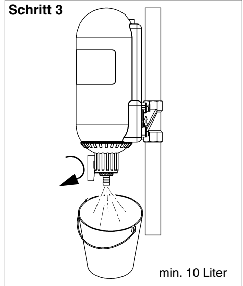
Abb. 8: Die Rückspülung wird gestartet indem der Spülhahn aufgedreht wird. Ein Auffanggefäß mit min. 10 Liter Volumen bereitstellen. Vorsicht Heißwasser, Verbrühungsgefahr!
