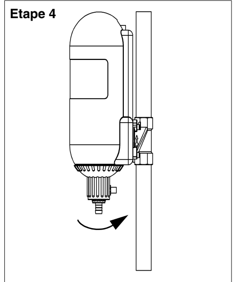
Fig. 9: Lorsque la performance du rétro lavage est terminée, fermer le robinet à biseau sphérique et tourner en arrière. Ainsi l'appareil est de nouveau en position de service.
