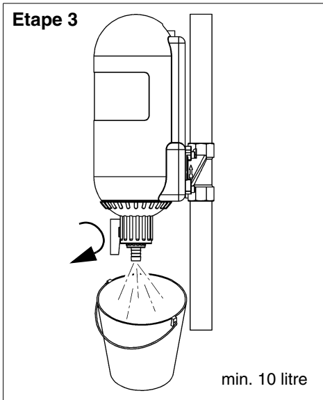
Fig. 7: Déclencher la performance du rétro lavage en ouvrant le robinet à biseau sphérique. Un réservoir collecteur / seau avec une capacité de minimum 10 litres doit être disponible. Attention EAU CHAUDE / Danger de brûlure.
