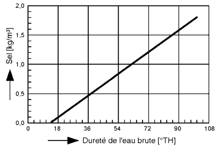
Fig. 6: Consommation de sel
