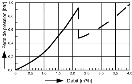
Fig. 4: Perte de pression
