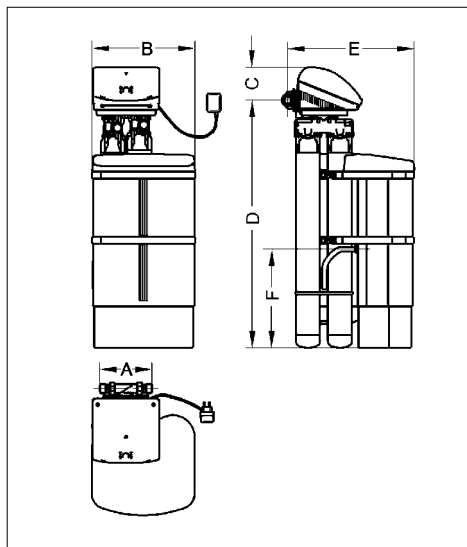
Fig. 2: Cotes de montage
