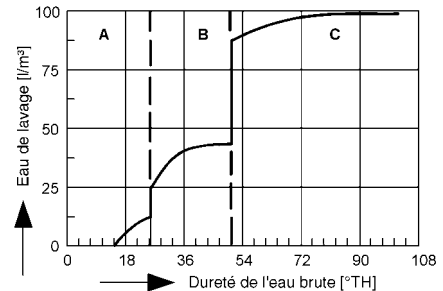
Fig. 7: Volume d'eau de lavage
