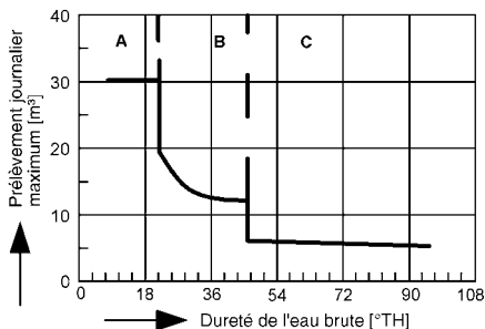
Fig. 5: Prélèvement journalier maximum
