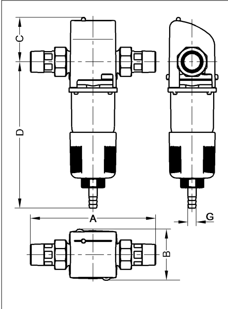
Fig. 6: Cotes de montage JEF-B ¾" - 1¼"
